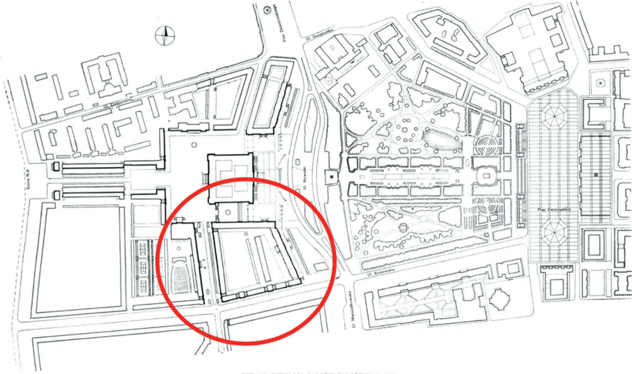
RYN. 423. SYTUACJA CAŁOŚCI ZAŁOŻENIA 1 : 4000
